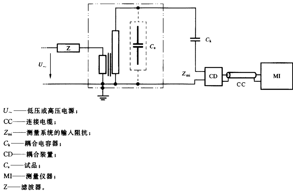
图 3 测量自激试品的试验回路
