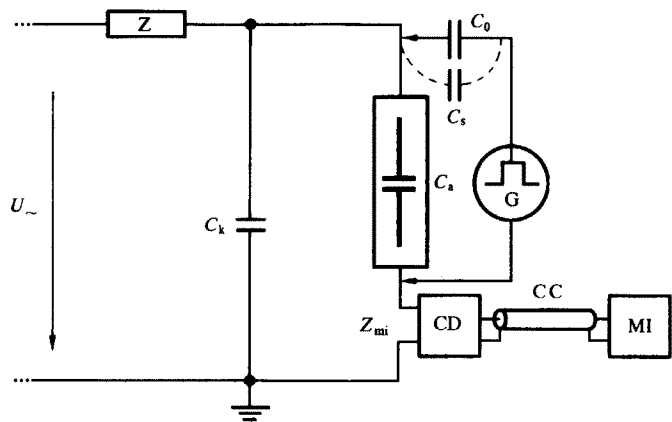
图 3 测量自激试品的试验回路
