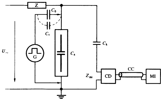
图 4 校准完整试验回路的接线
